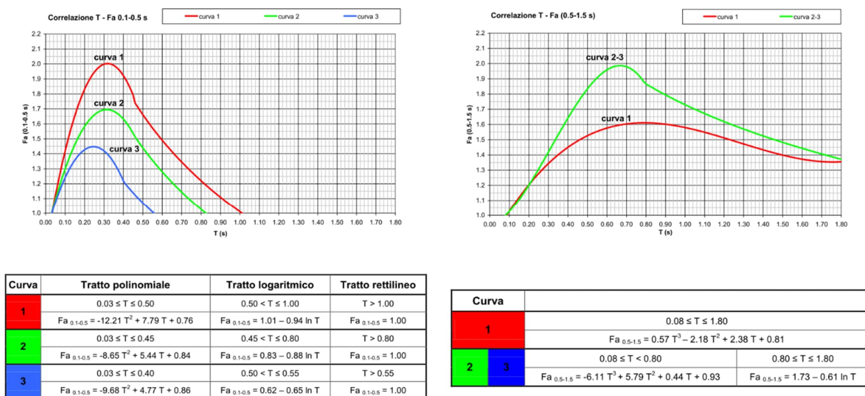
FIG. 28 – CURVE RAPPRESENTANTI I VALORI DI F_a AL VARIARE DAL PERIODO PROPRIO DEL SITO T PER LITOLOGIA SABBIOSA
