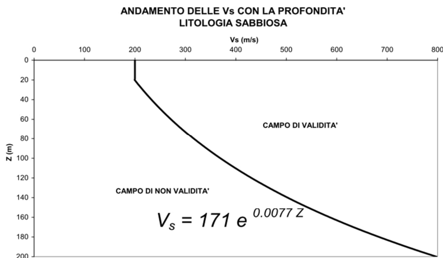
FIG. 26 – ANDAMENTO DELLE V_s IN FUNZIONE DELLA PROFONDITÀ PER LA LITOLOGIA SABBIOSA
