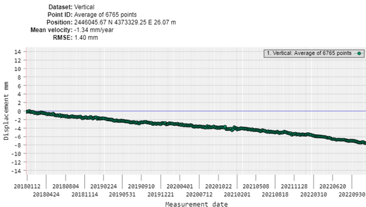
FIG. 7 – GRAFICO DERIVANTE DALLE MISURE INTERFEROMETRICHE RELATIVE A 6765 PUNTI UBICATI PRESSO L'AREA DI STUDIO
