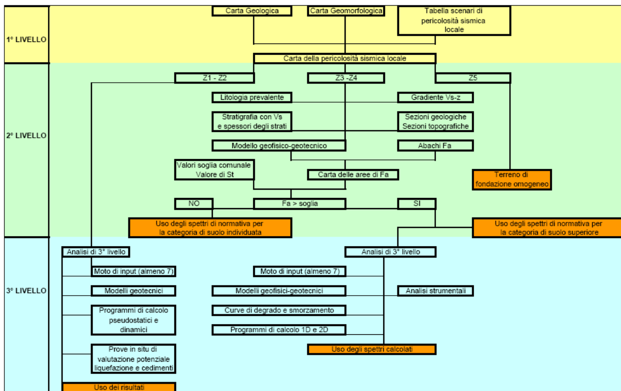
FIG. 25 – DIAGRAMMA DI FLUSSO DEI DATI NECESSARI E DEI PERCORSI DA SEGUIRE NEI TRE LIVELLI DI INDAGINE
