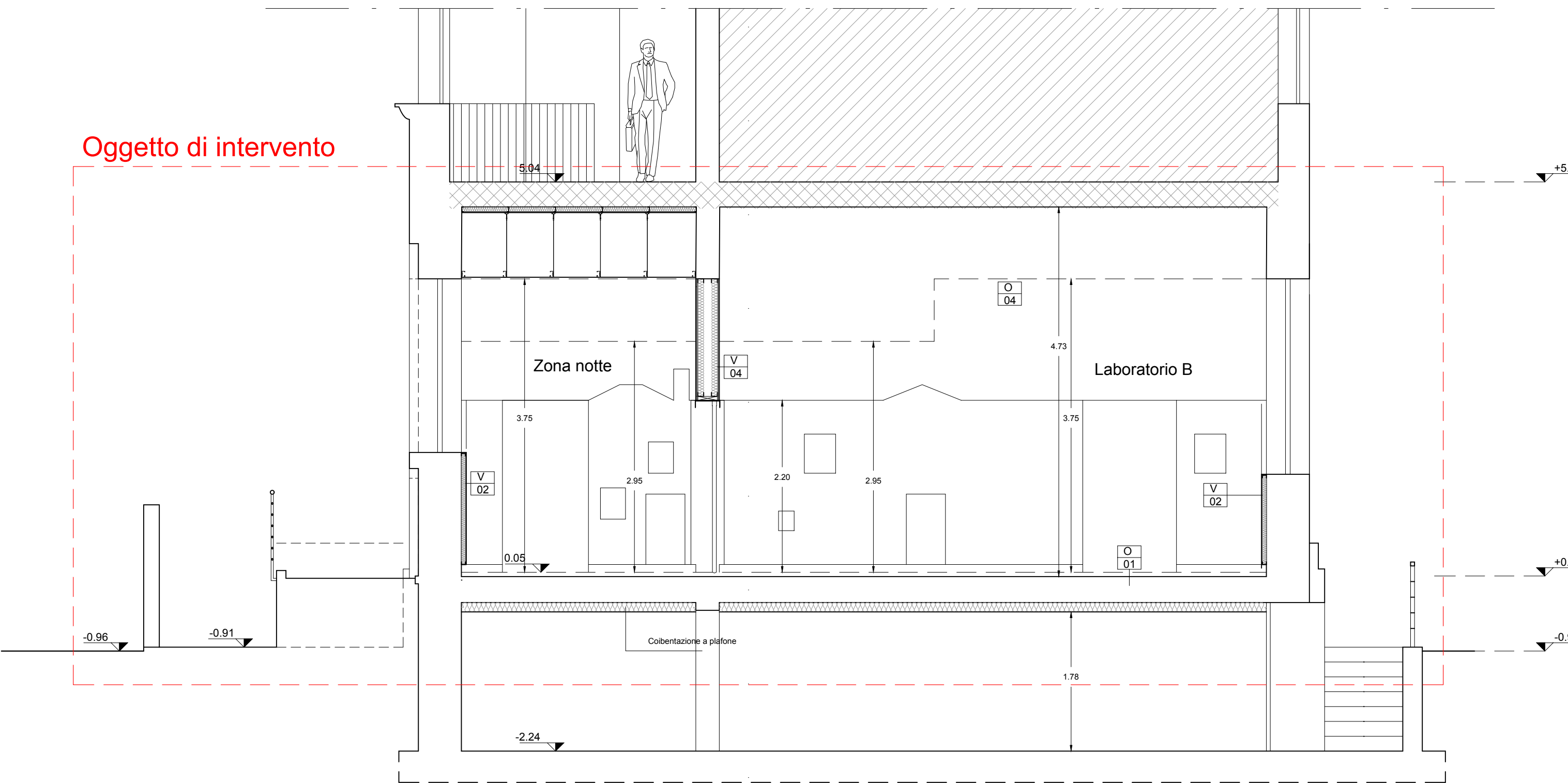
SEZIONE D-D
