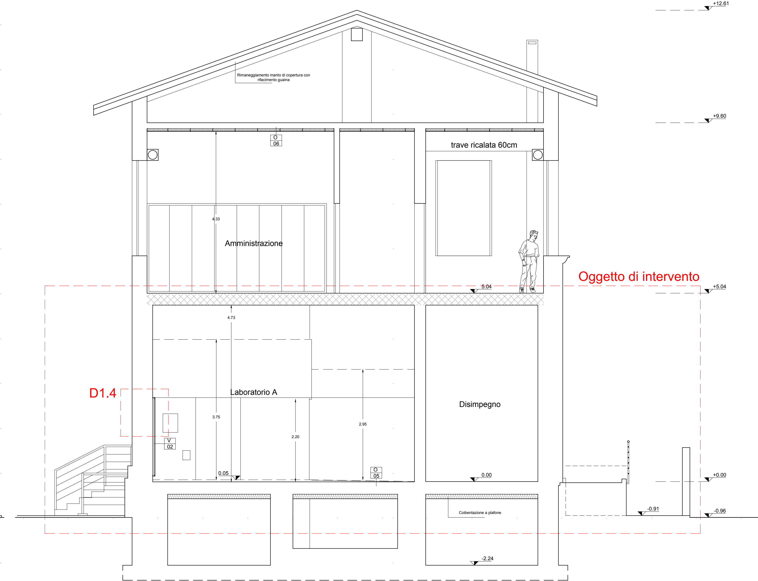
SEZIONE C-C
