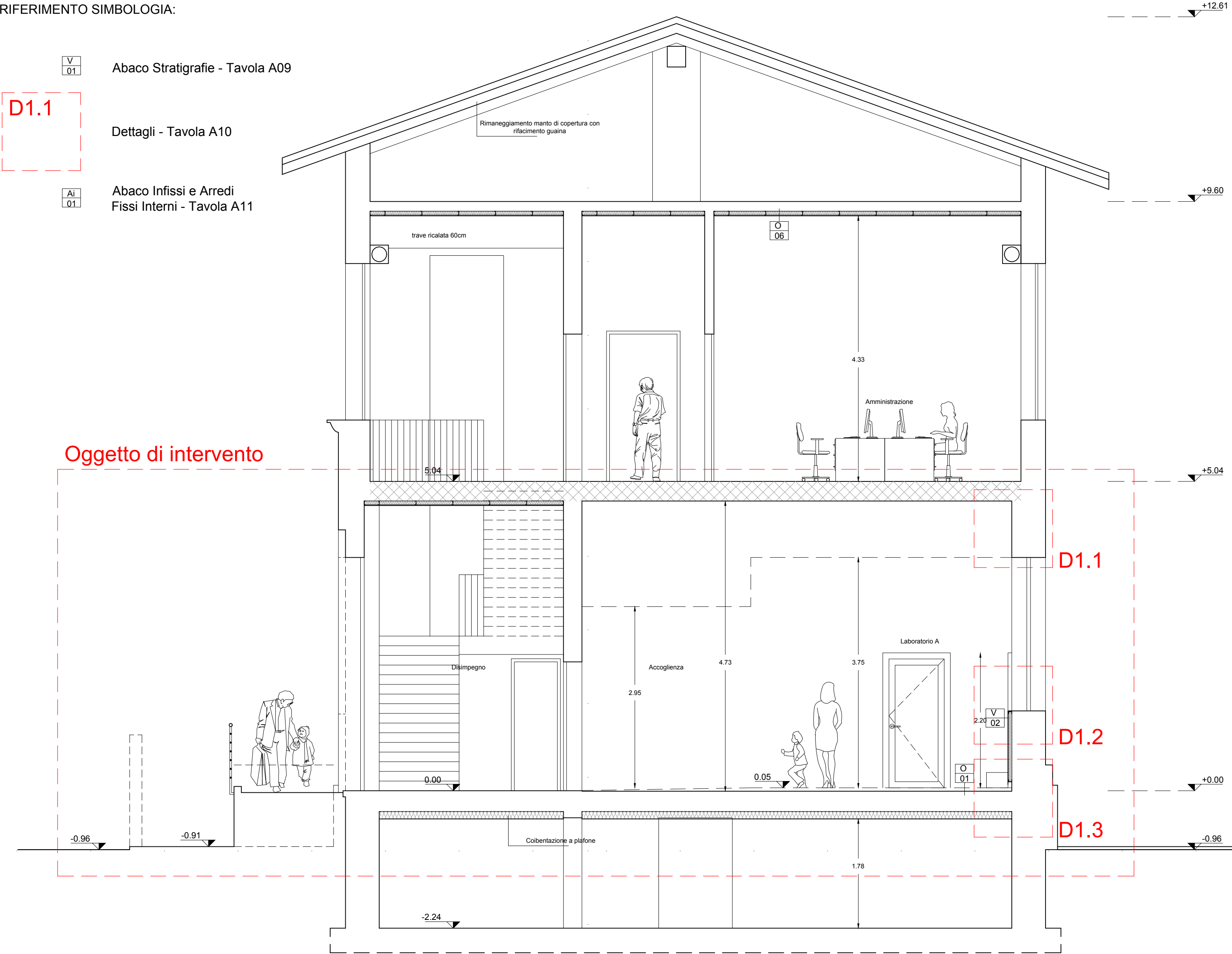
SEZIONE B-B
