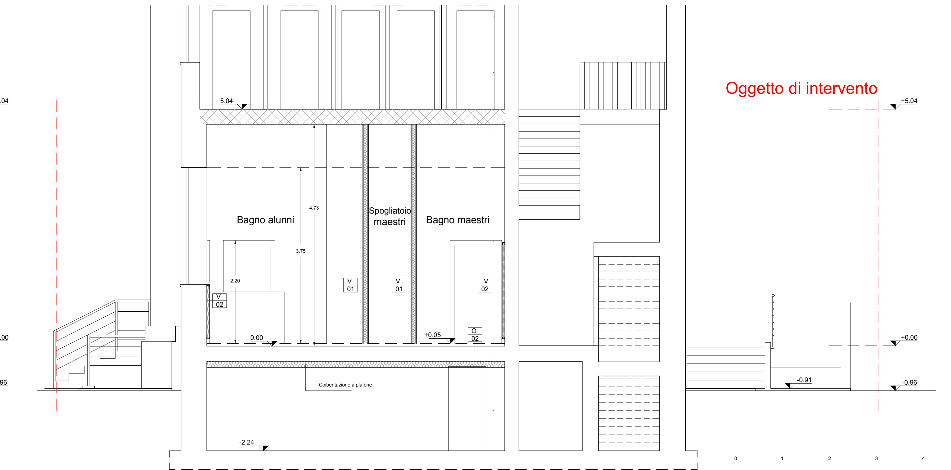
SEZIONE E-E
