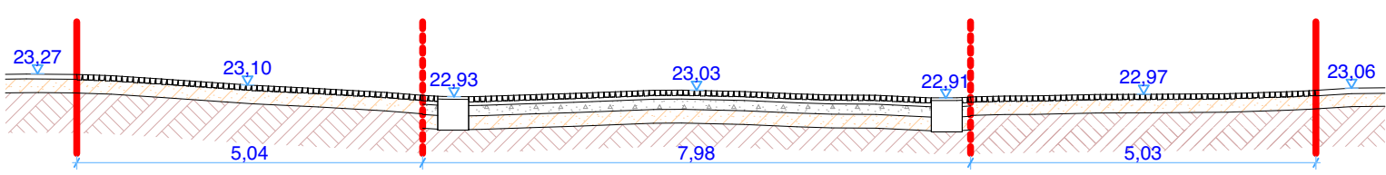
SEZIONE 02 Scala 1:100
